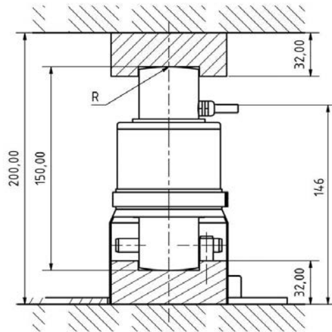
Dimensiones (mm)
