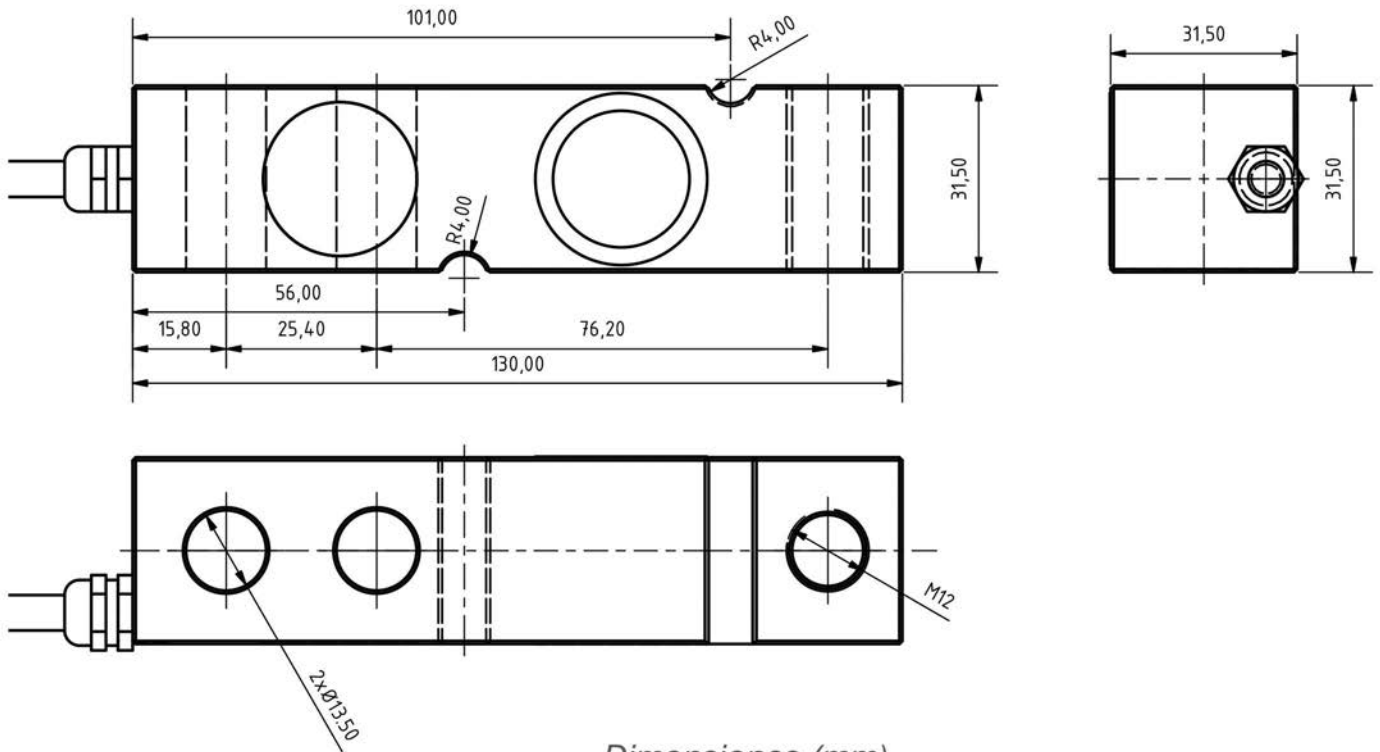
Dimensiones (mm)
